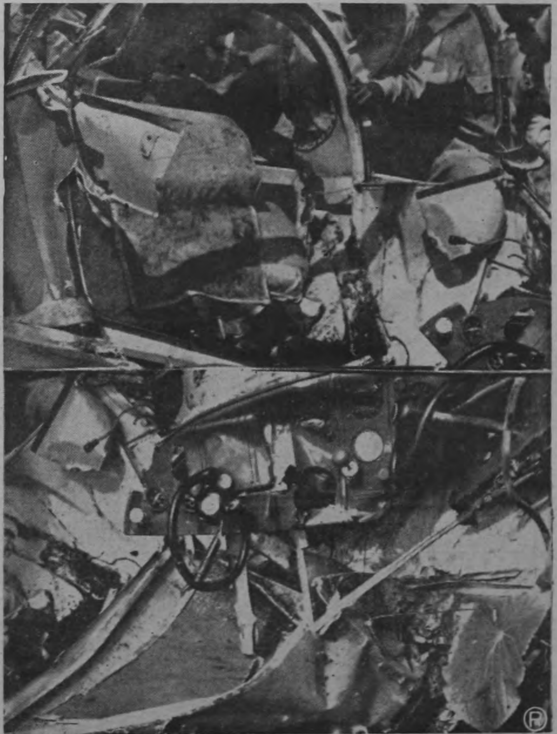
ARRIBA: Vista de los restos de la parte trasera de la cabina del Ercoupe TI-254. En este sitio se presume viajaban la señora Emilia Castro Silvia de Barish y sus dos pequeños hijos, quienes salieron despedidos a través del plástico y metal, cayendo a varios metros del avión destrozado al chocar con un grueso tronco que despedazó el frágil aparato.
